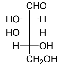
D-lyxose
