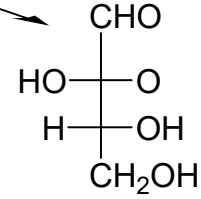
D-threose
