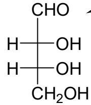
D-erythrose
