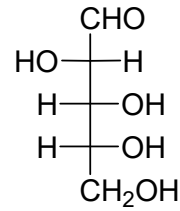
D-arabinose
