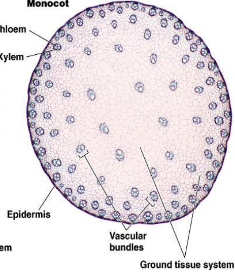
Monocot
