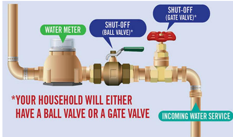
الشكل (7): يوضح نموذج لمحبس ماء رئيسي .
