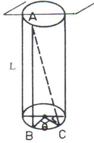
الشكل (13) حساب ثابت الليّ
