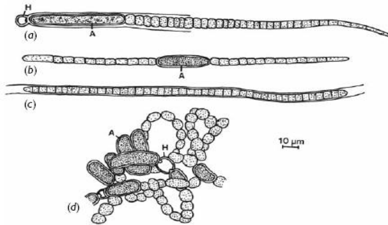
Fig. 2.18 (a) Gloeotrichia echinulata . (b) Aphanizomenon flos-aquae . (c) Phormidium inundatum . (d) Anabaena flos-aquae . (A) Akinete; (H) heterocyst. (After Prescott, 1962.)
