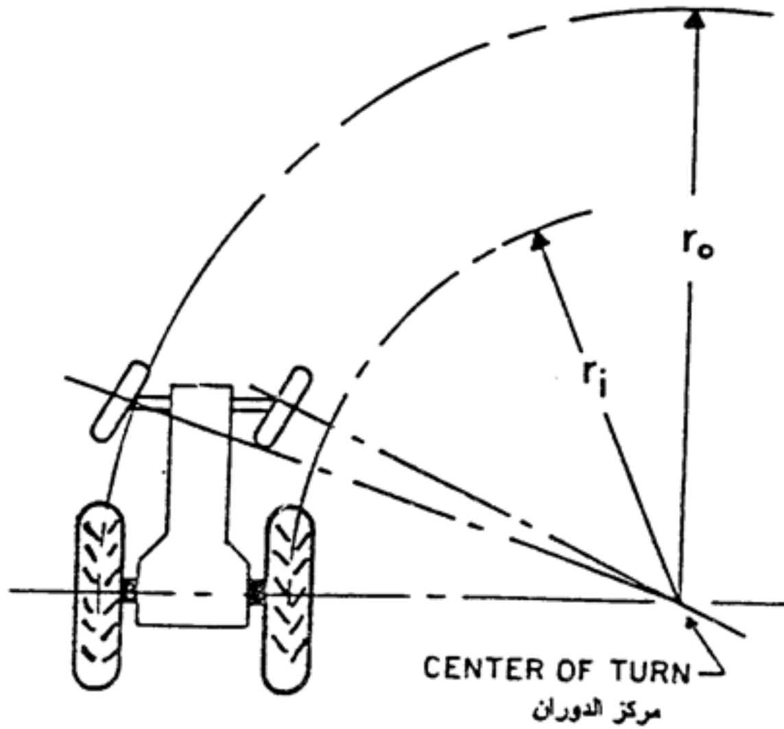
شكل (١٩-٤) سير الجرار في منحنى
