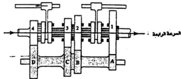
شكل (٤-١٠): تغيير السرعات في صندوق التروس
