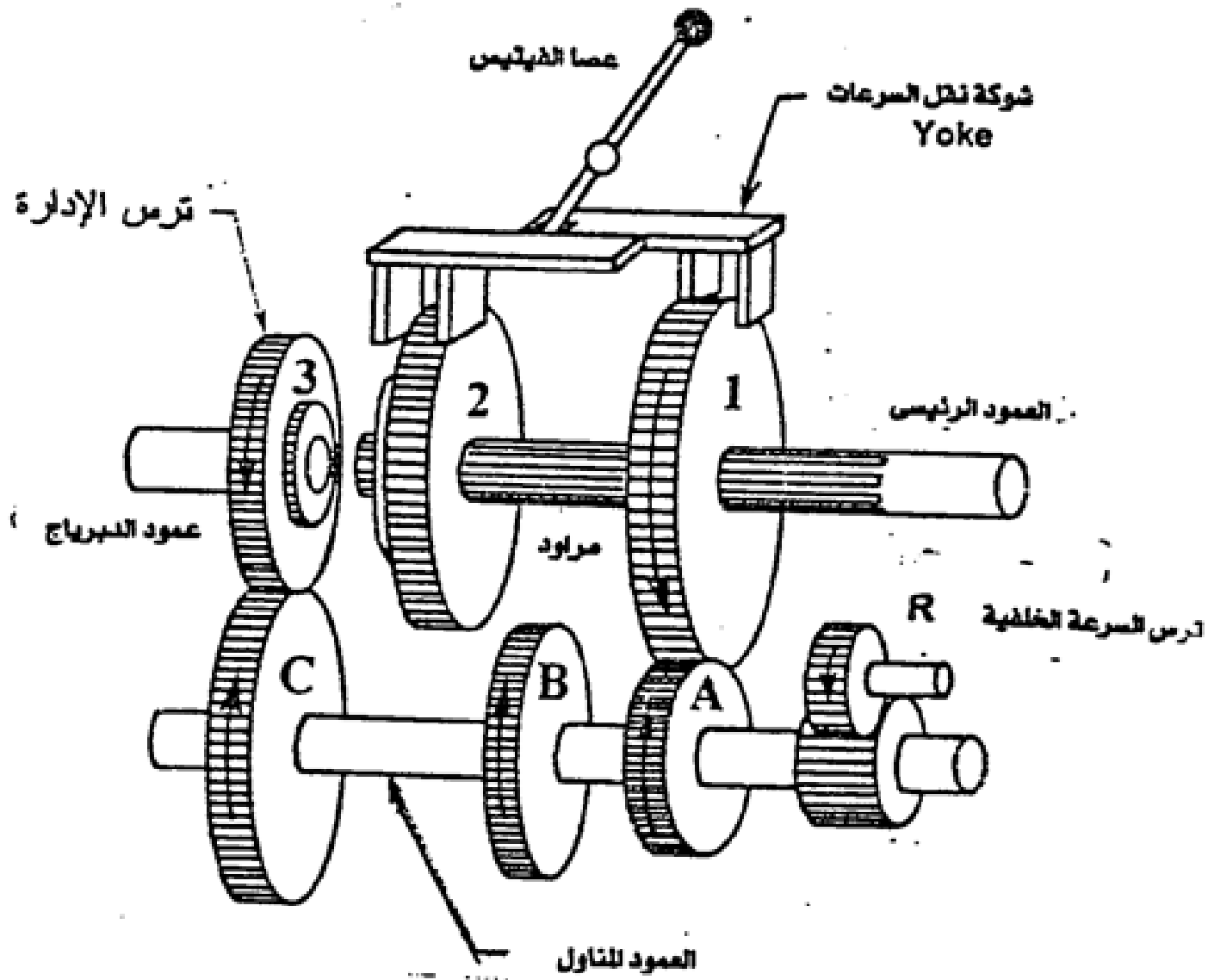
شكل (٤-٨) صندوق التروس المنزقة
