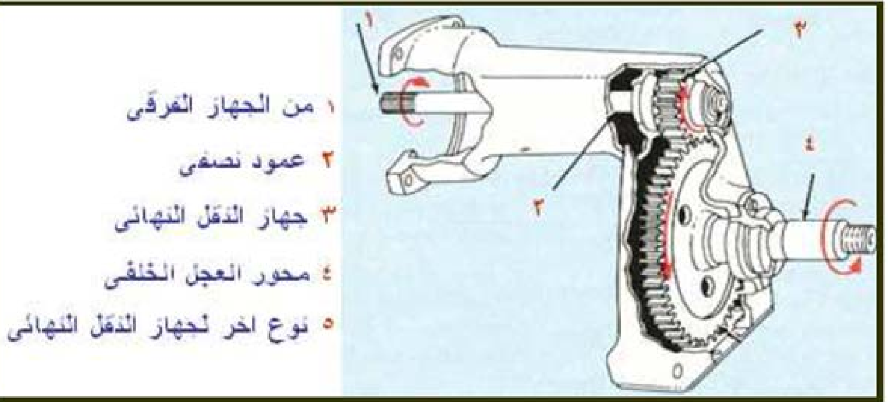
شكل ( ) : جهاز النقل النهائي
