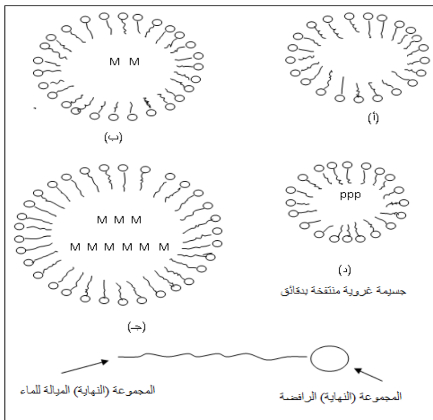
شكل - 1 - اشكال تخطيطية تمثل البلمرة في الوسط المستحلب
