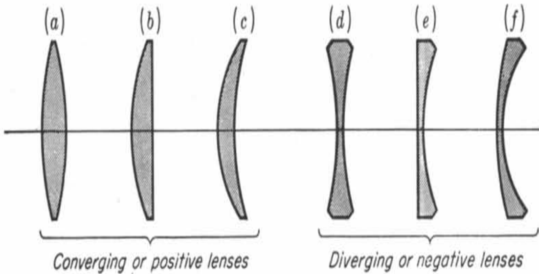
الشكل (1) مجموعة العدسات اللامة والمفرفة
