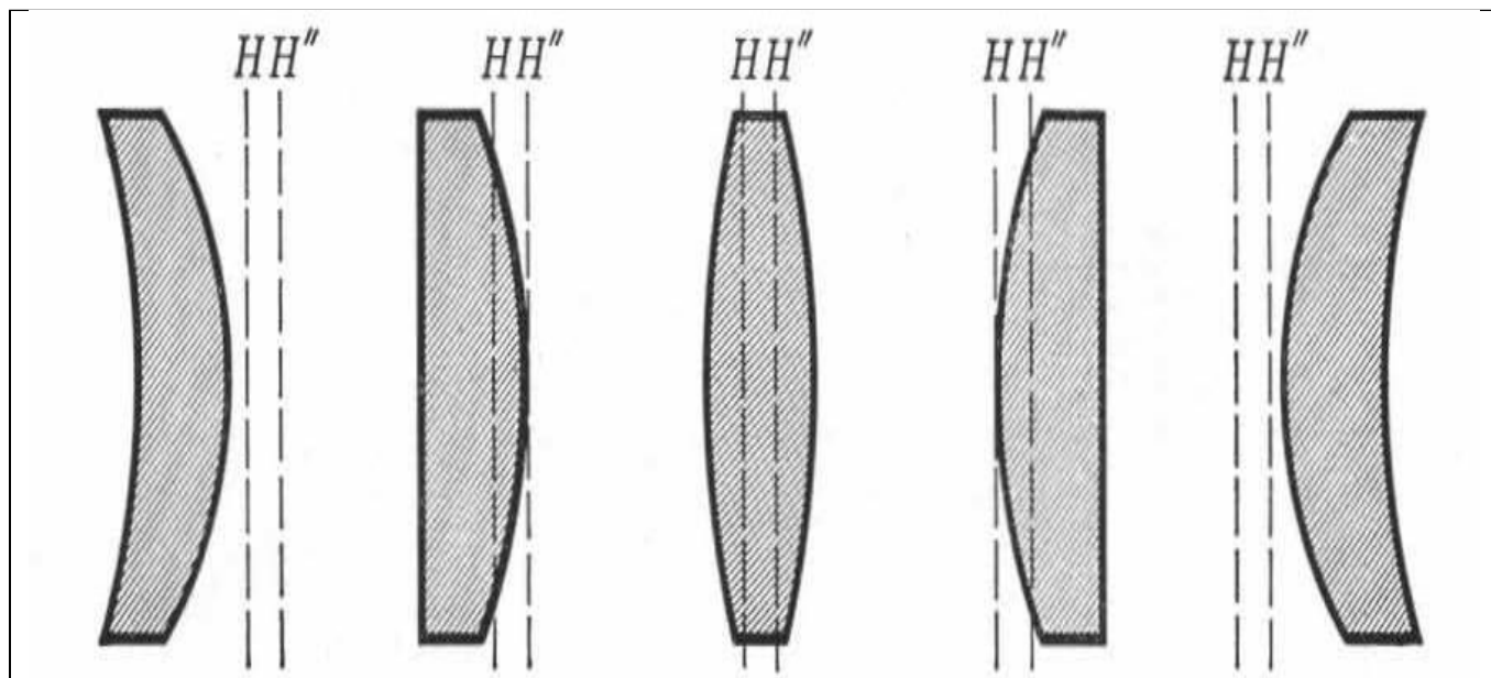
الشكل (6) : موقع النقاط الأساسية بالنسبة لأنواع العدسات السمكية
