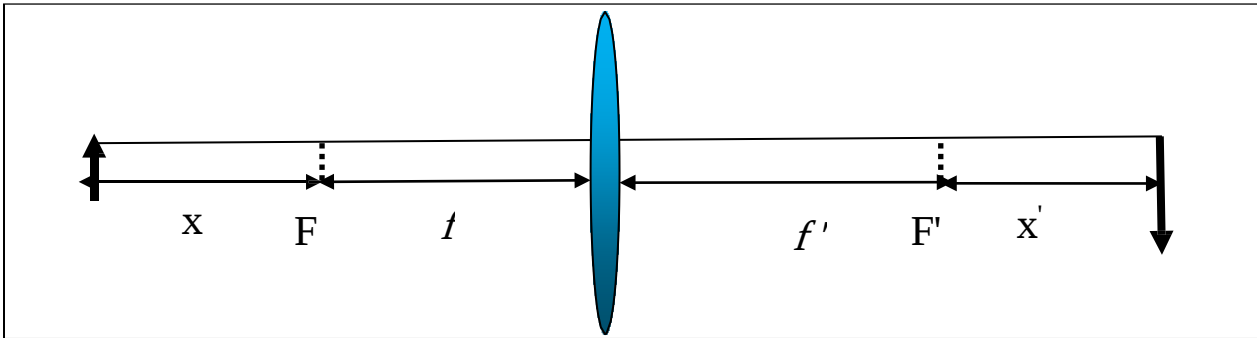
الشكل (4) : الابعاد البصرية لصيغة نيوتن للعدسات
