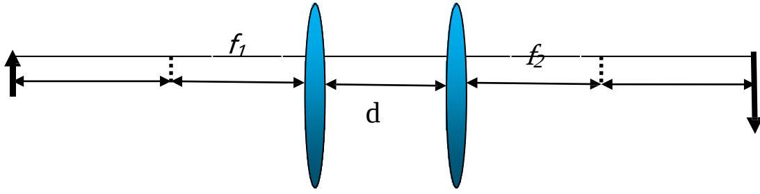
الشكل (3) : العدسة المركبة
